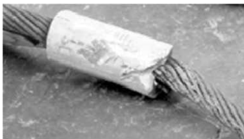
איור 7. נזק לשרוול אלומיניום
