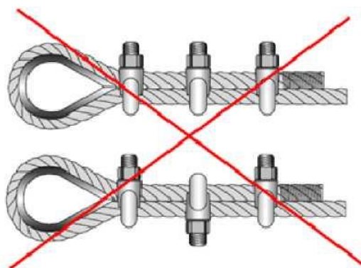
איור 10. חיבור קצה עם חבקי חבל שהותאמו בצורה לא נכונה
