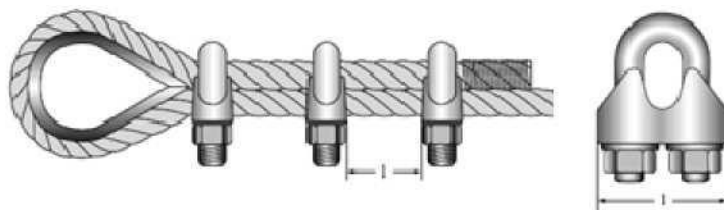
איור 9. כיוון נכון לחבקי חבלים
